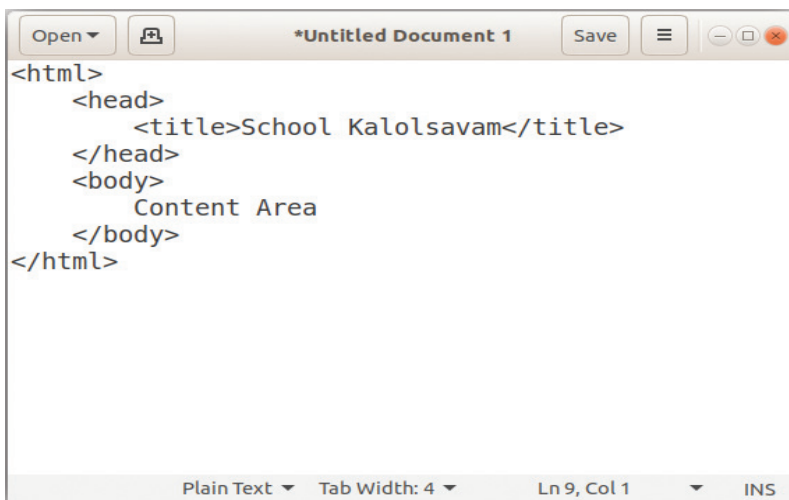
Fig. 8.3 Basic HTML tags
